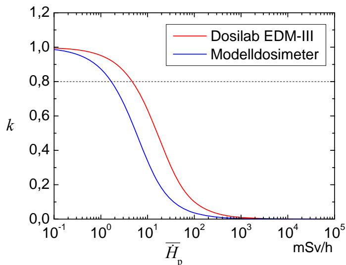
Abb. 16 Relatives Ansprechvermögen k im Strahlungsfeld eines medizinischen Therapiebeschleunigers in Abhängigkeit der mittleren Dosisleistung.
