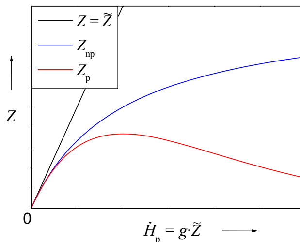
Abb. 2 Schematische Abhängigkeit der Zählrate Z von der Personendosisleistung \dot{H}_p bei paralyisierendem (p) und nichtparalyisierendem (np) Totzeitverhalten.
