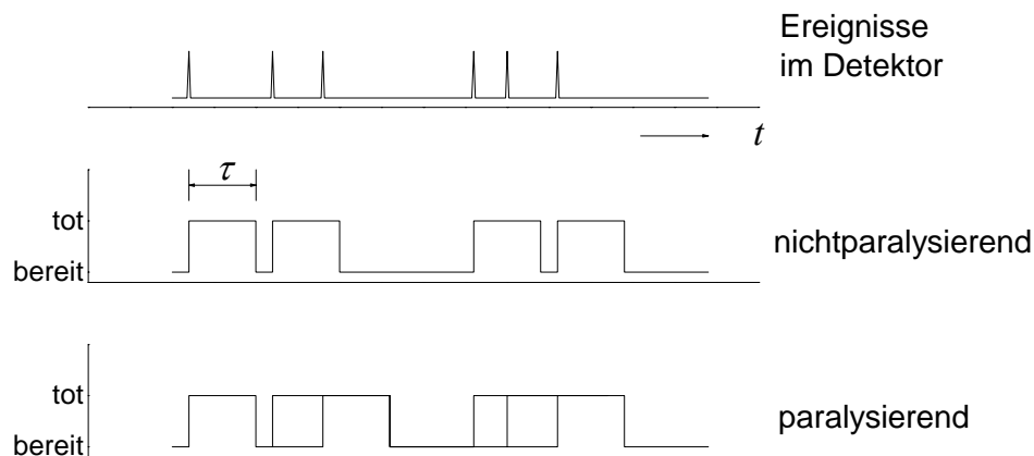
Abb. 1 Paralyisierendes und nichtparalyisierendes Totzeitverhalten von Strahlungsdetektoren
