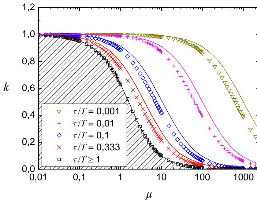
Abb. 9 Relatives Ansprechvermögen bei sinusförmiger Pulsform für verschiedene Totzeiten. Die durchgezogenen Linien entsprechen dem Ansprechvermögen für jeweils gleichbreite und flächengleiche Rechteckpulse.
