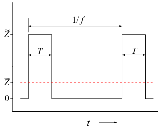
Abb. 4 Parameter der untersuchten Rechteckpulsung.
