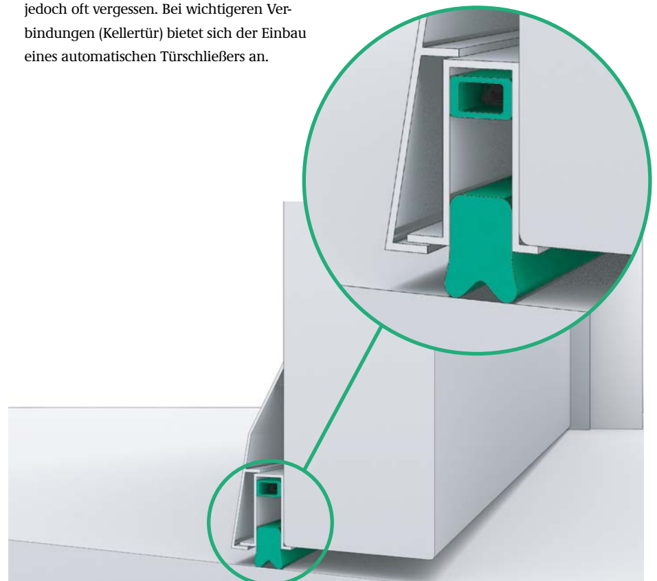
Abb. 7.13: Bewegliche Anpress-Schwelldichtung
